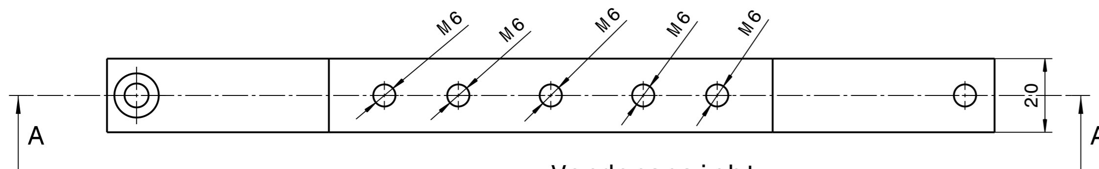
Vorderansicht Maßstab: 1:1
